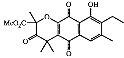
annulin B
